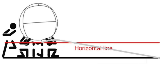
図4 有効な軌道のヒット
